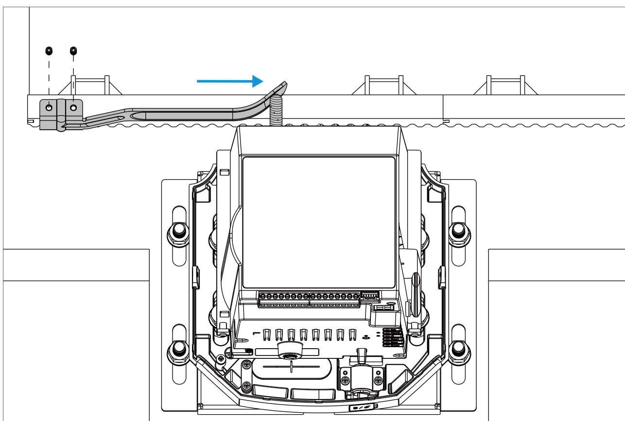
Fixez la tôle de butée gauche
